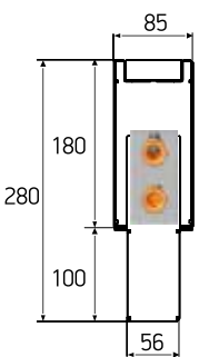
KPZ 85-180-xxxx.00.000-01
