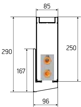
KPZ 85-250-xxxx.00.000-01-2/C
