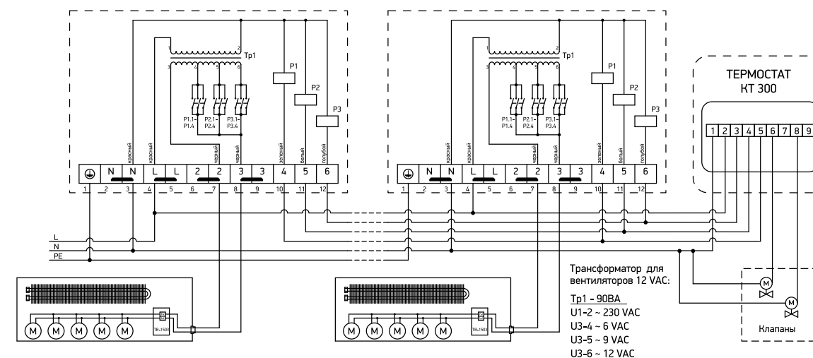
Рис. 1. Схема подключения конвекторов с питанием 12В к термостату Techno KT 300 с трёхступенчатой регулировкой скорости вращения вентиляторов с помощью блоков BRT 90.
