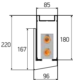
KPZ 85-180-xxxx.00.000-01/C
