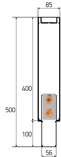
KPZ 85-400-xxxx.00.000-01-2
