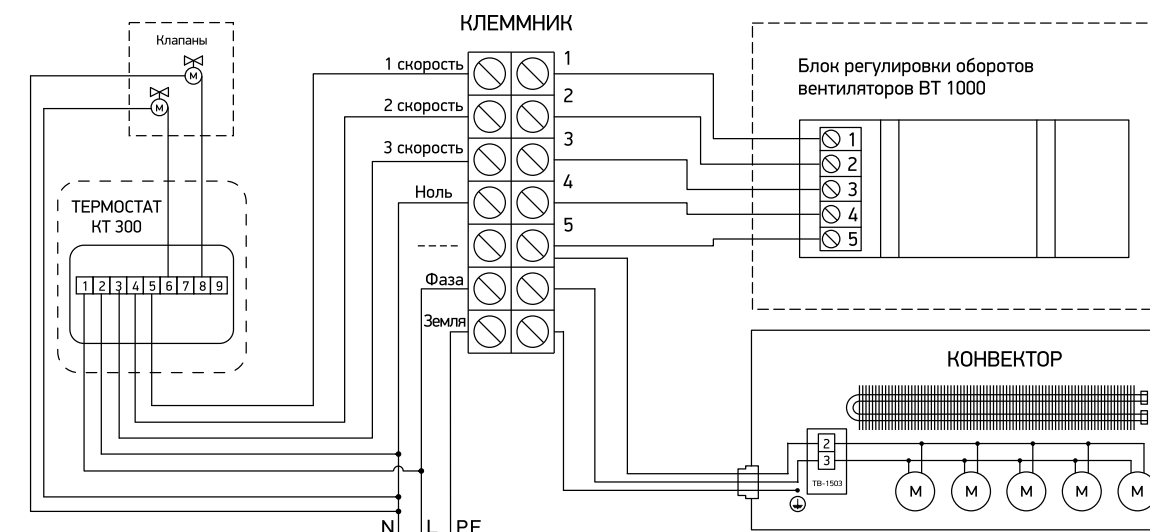
Рис. 3. Схема подключения конвекторов с питанием 220В к термостату Techno KT 300 с трёхступенчатой регулировкой скорости вращения вентиляторов с помощью блока BT-1000.
