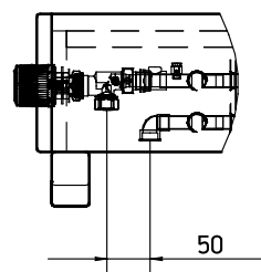
С терморегулятором
