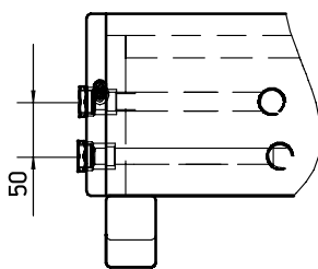
Сбоку
